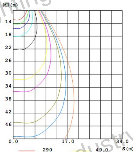
垂直照度図
