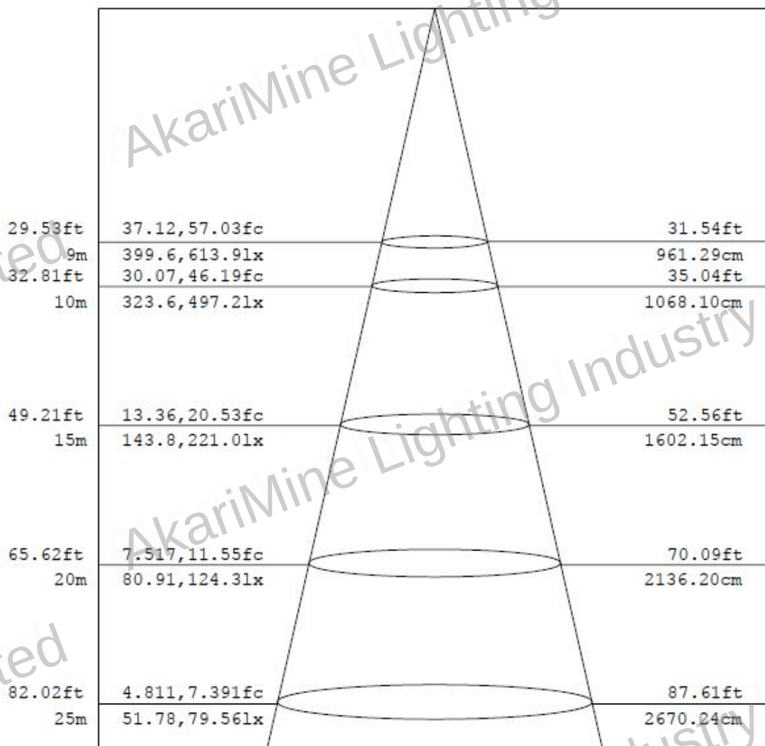
垂直照度図
